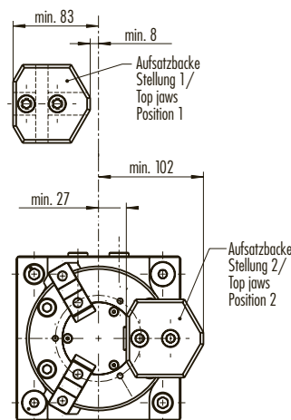
Draufsicht - Top view
