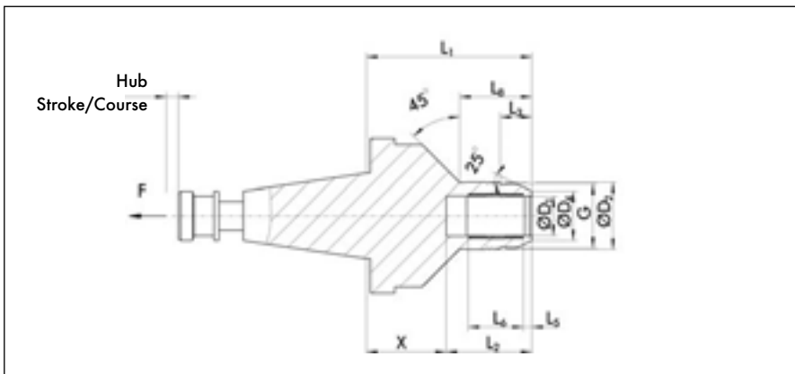
Zwischenbüchsen-sicherung mit Überwurfmutter Locking of intermediate sleeve with cap nut
